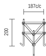
A132 - Bolt Cage
