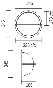
C313G - Brenton 1 Arm
