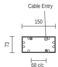
Mini Serengeti Back Plate Detail
