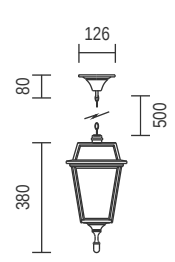
T109E - Chain Hanging
