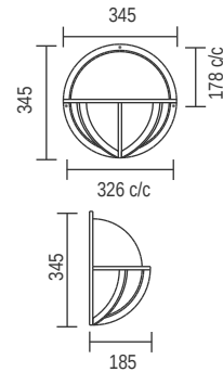
C315G - Brenton 4 Arm
