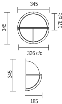
C314G - Brenton 2 Arm
