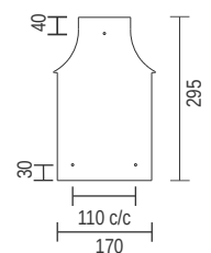
Mini Empire Back Plate Detail
